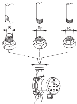
Obr. 26 Závít G a závít R
